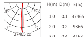
XP-E2 7° 2200K
