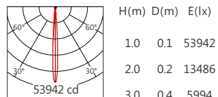
XP-E2 7° 3000K
